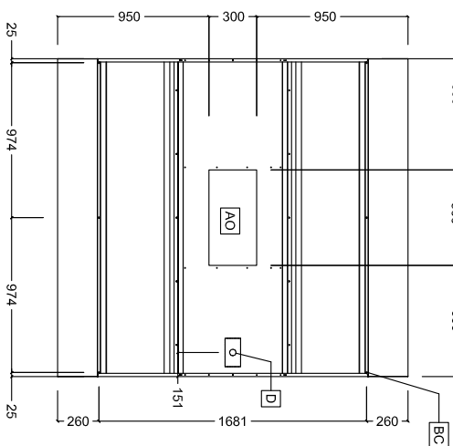
Felülnézet
